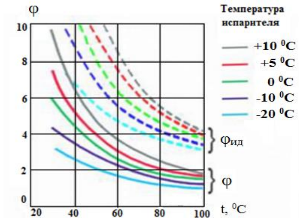
Рис. 2. Идеальный и действительный коэффициент преобразования тепловых насосов с поршневым компрессором
