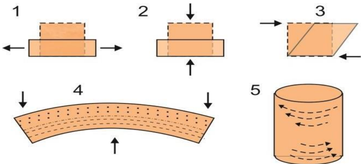
2.2 - rasm. Ayrim turdagi deformatsiyalar va ta'sir kuchlarning yo'nalishlari (1 - cho'zilish, 2 - siqilish, 3 - siljish, 4 - bukilish, 5 - aylanma)
