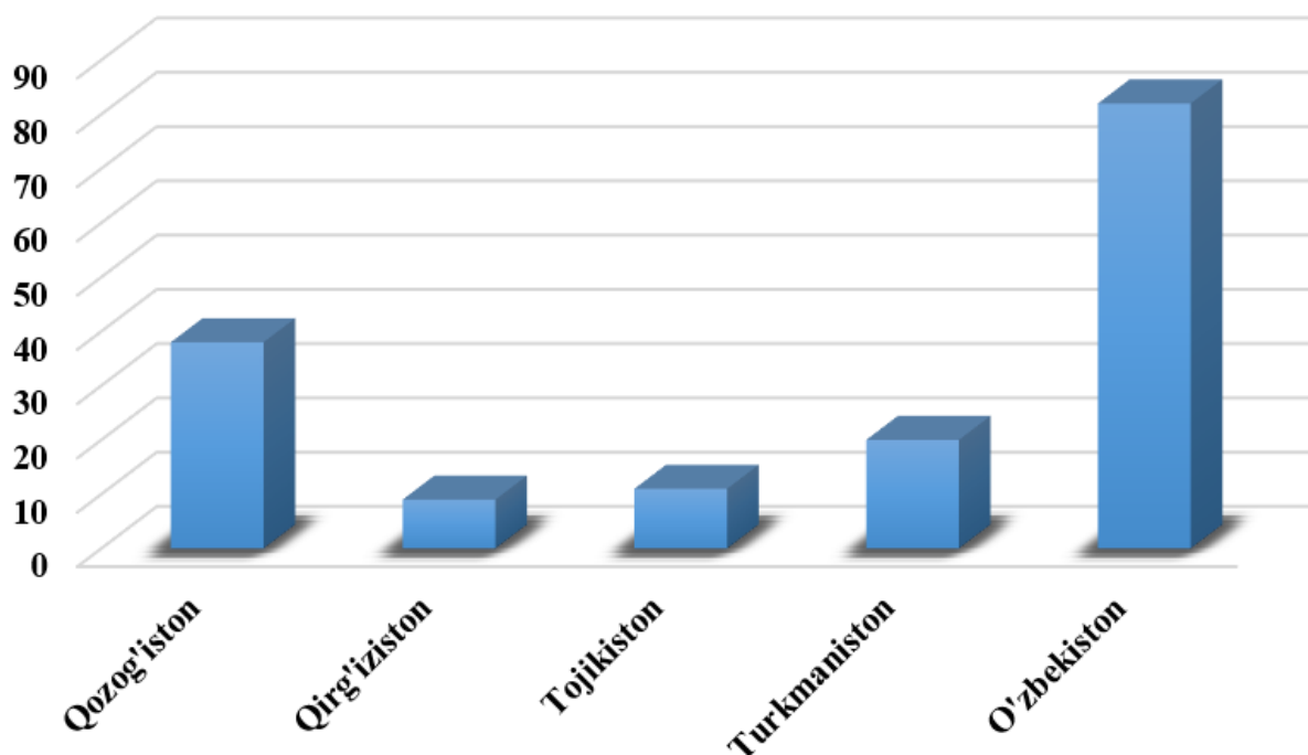
1-rasm. O'rtasiy mintaqasida chuchuk suvdan foydalanish hajmi, kub.km/yil.
