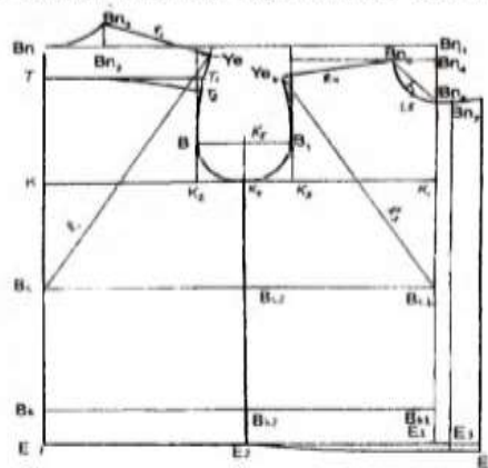
62-rasm. Erkaklar ko'ylagining chizmasi
